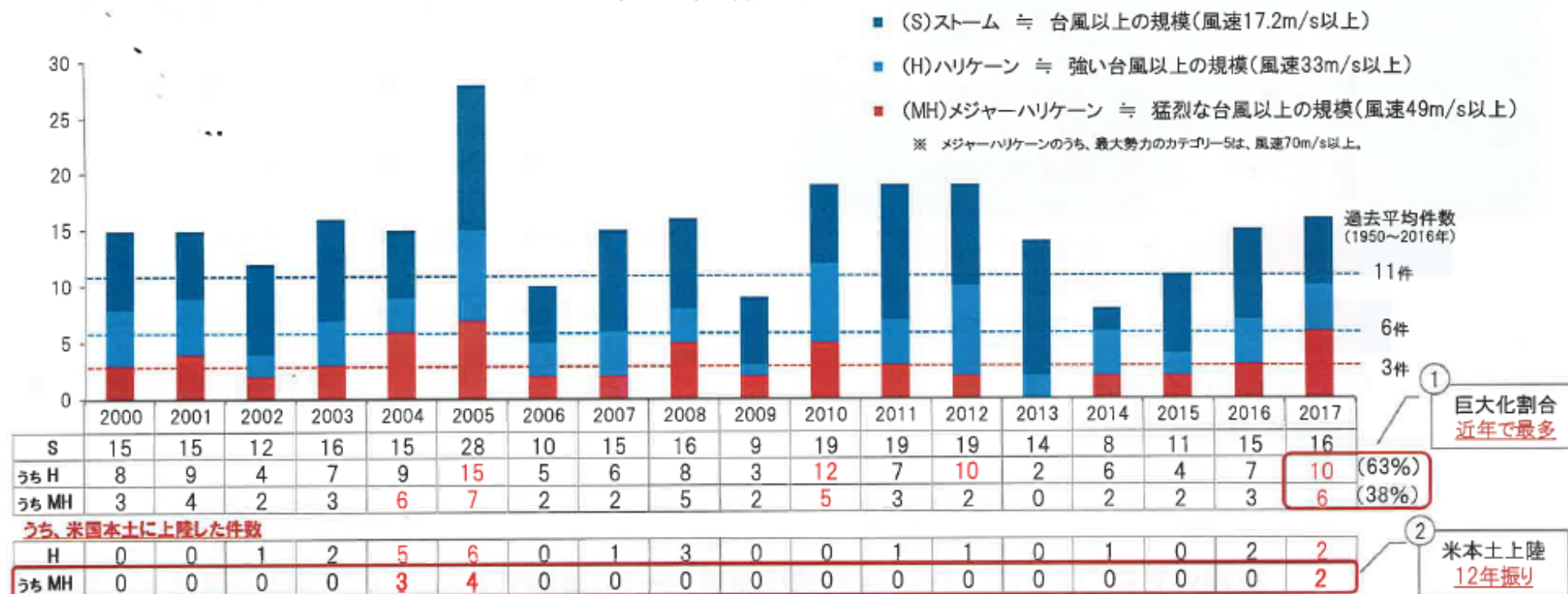
ストーム以上の勢力に拡大した風害の発生件数と上陸件数の推移 (2000年以降)
