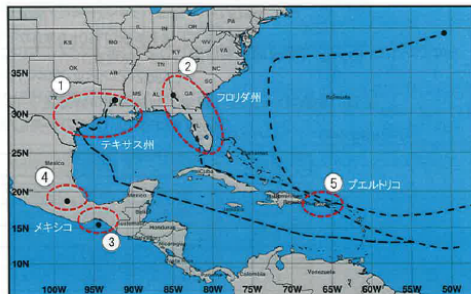
ハリケーン進路と地震発生地域
