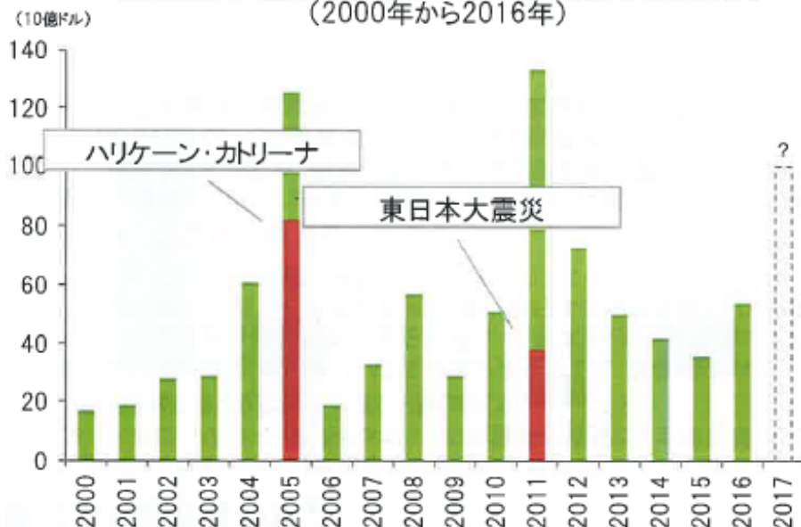
各年の自然災害による保険業界損失額の推移
